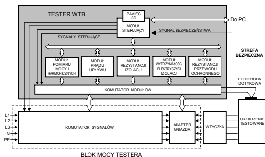
Rys. 2. Schemat połączenia testera z blokiem mocy obciążonym obiektem badań
